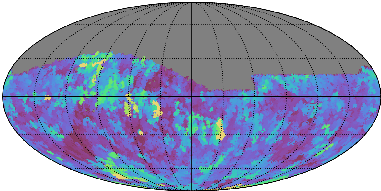
weather_cloudso20v3.4_10yrs Yr 1 z band: Max seeingGeom
