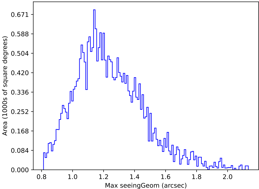
weather_cloudso20v3.4_10yrs Yr 1 z band: Max seeingGeom
