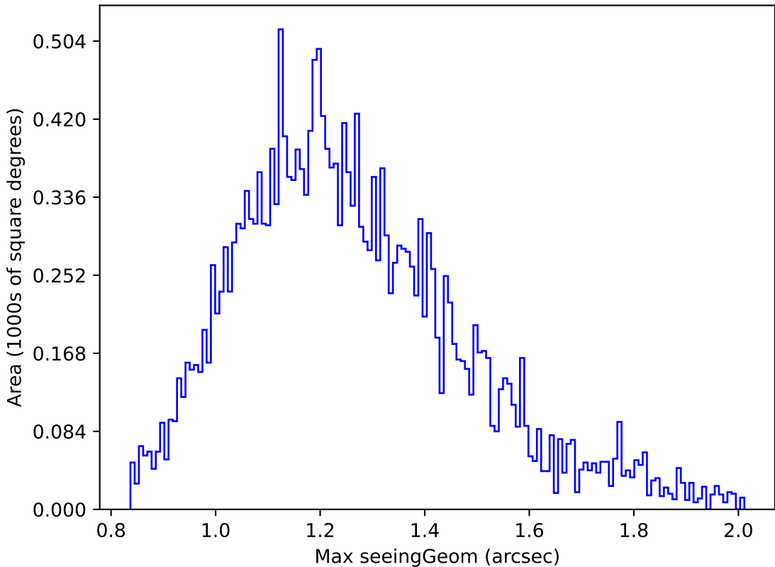
weather_cloudso20v3.4_10yrs Yr 1 y band: Max seeingGeom
