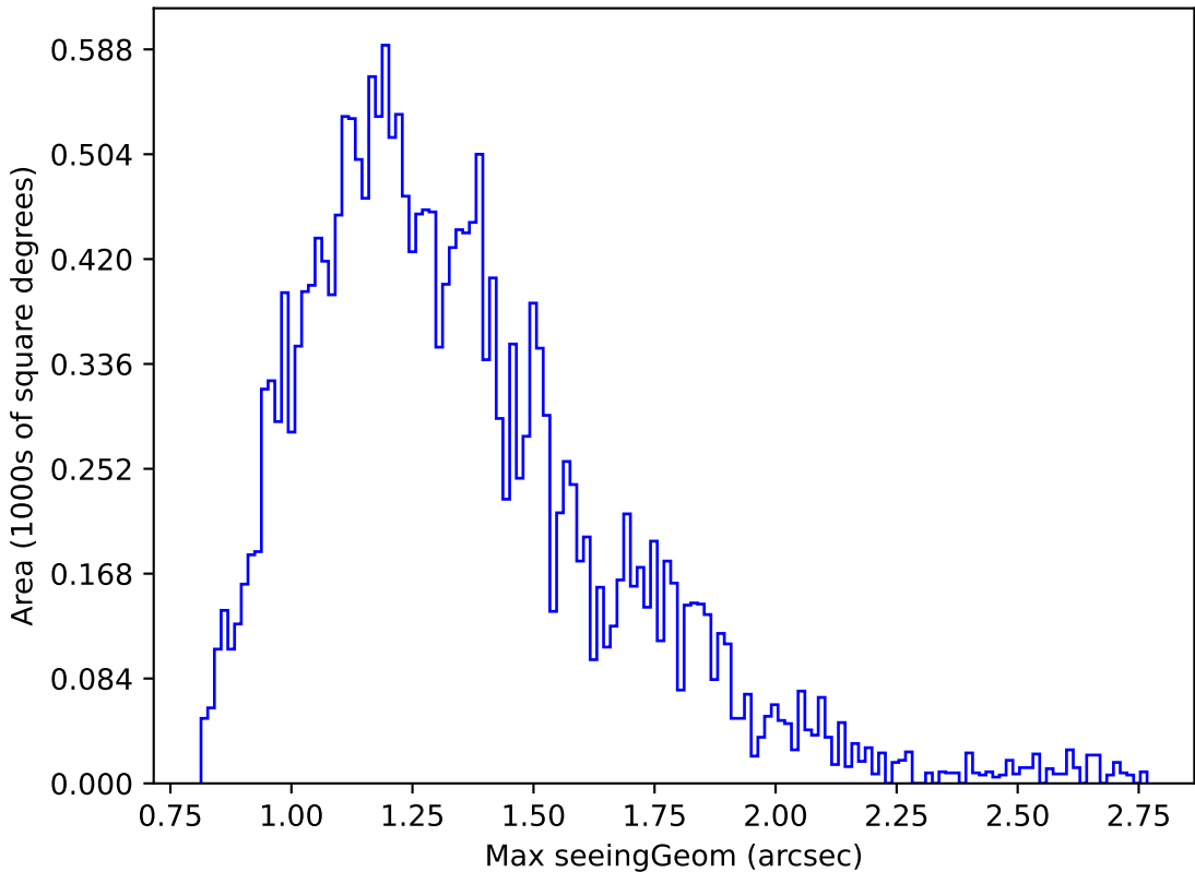
weather_cloudso20v3.4_10yrs Yr 1 u band: Max seeingGeom
