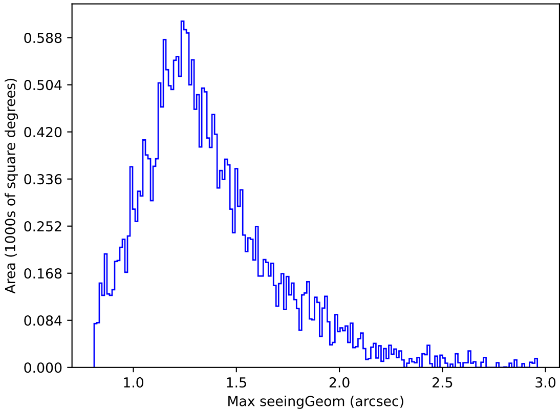
weather_cloudso20v3.4_10yrs Yr 1 r band: Max seeingGeom
