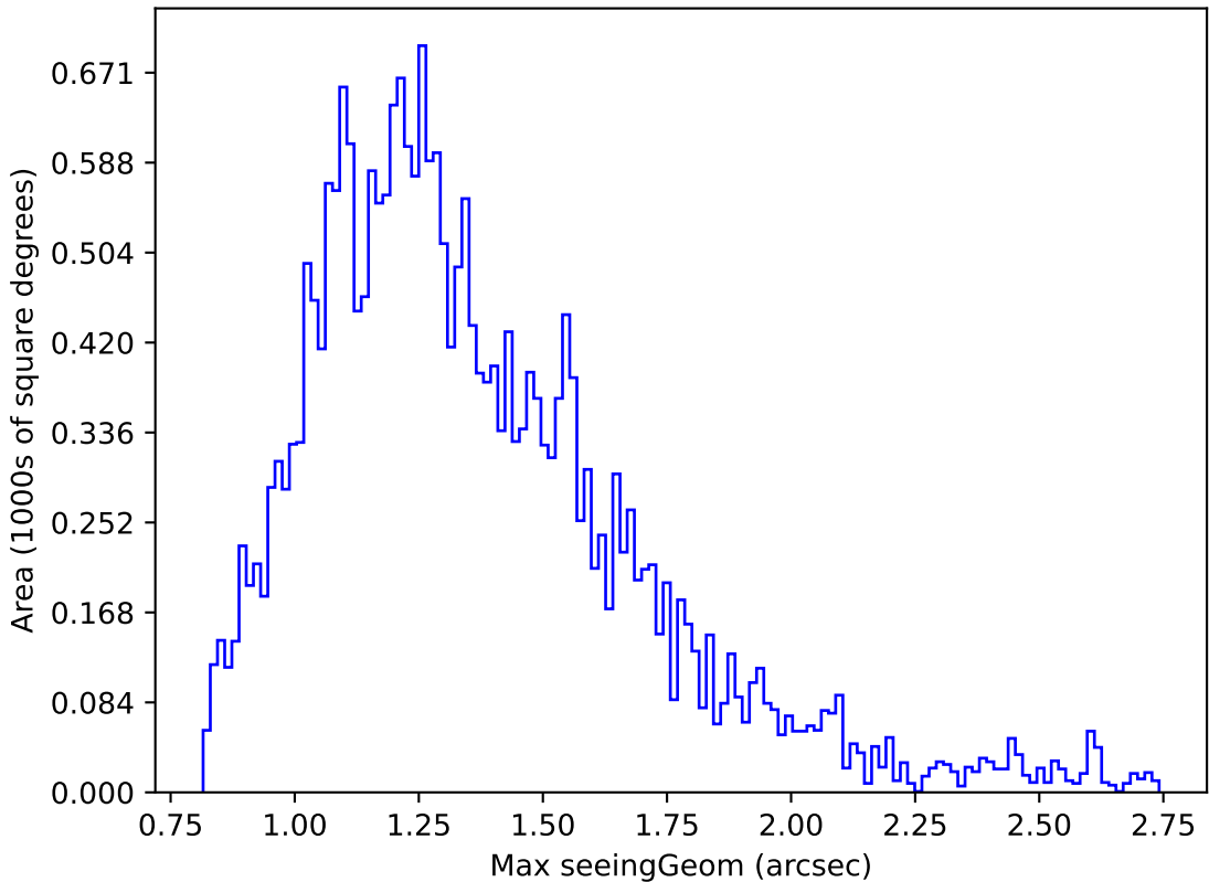
weather_cloudso20v3.4_10yrs Yr 1 i band: Max seeingGeom
