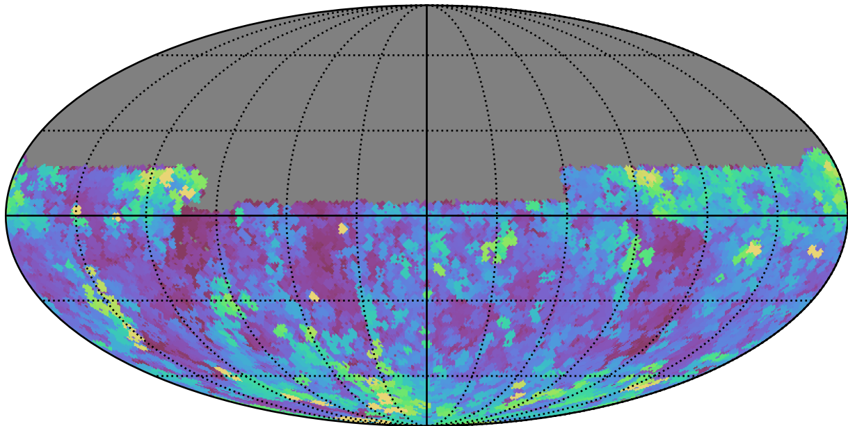
weather_cloudso20v3.4_10yrs Yr 1 y band: Max seeingEff
