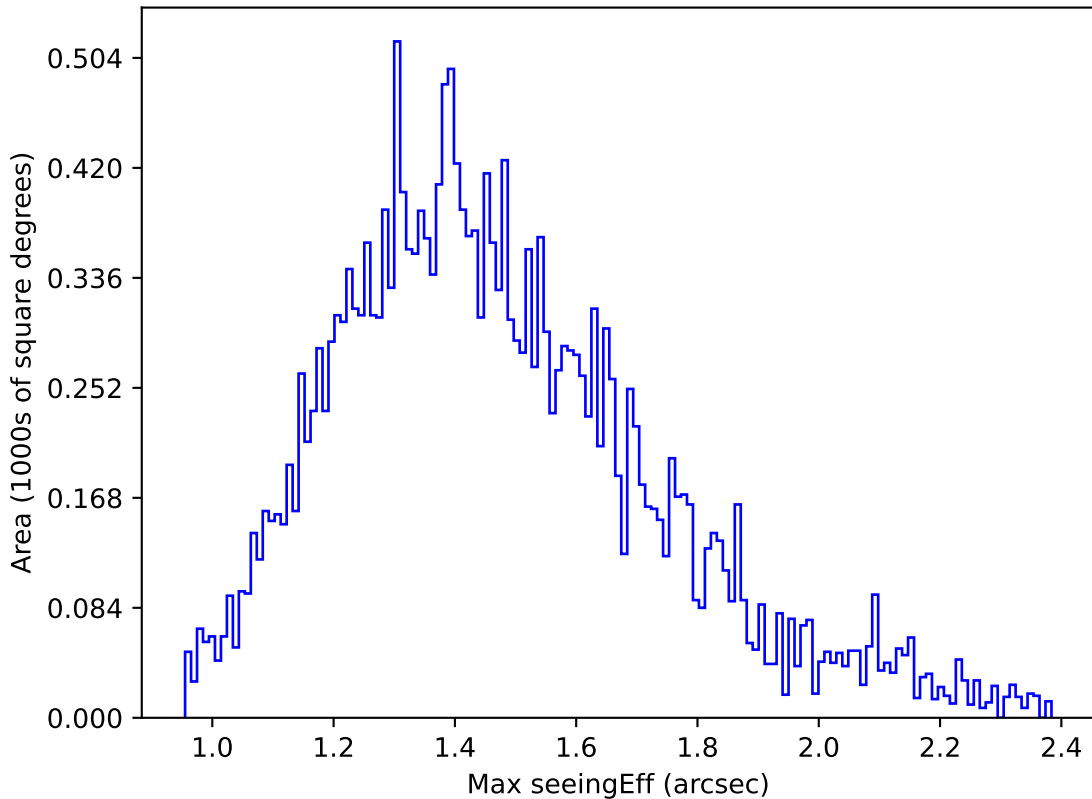
weather_cloudso20v3.4_10yrs Yr 1 y band: Max seeingEff
