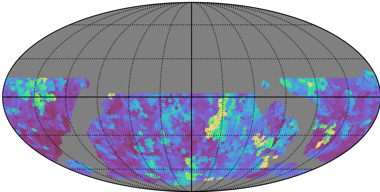
weather_cloudso20v3.4_10yrs WFD z band: Max seeingEff
