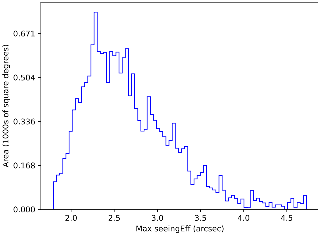
weather_cloudso20v3.4_10yrs WFD z band: Max seeingEff
