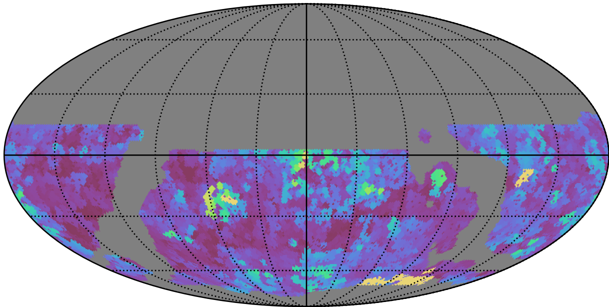
weather_cloudso20v3.4_10yrs WFD y band: Max seeingEff
