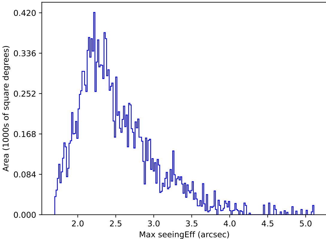
weather_cloudso20v3.4_10yrs WFD y band: Max seeingEff
