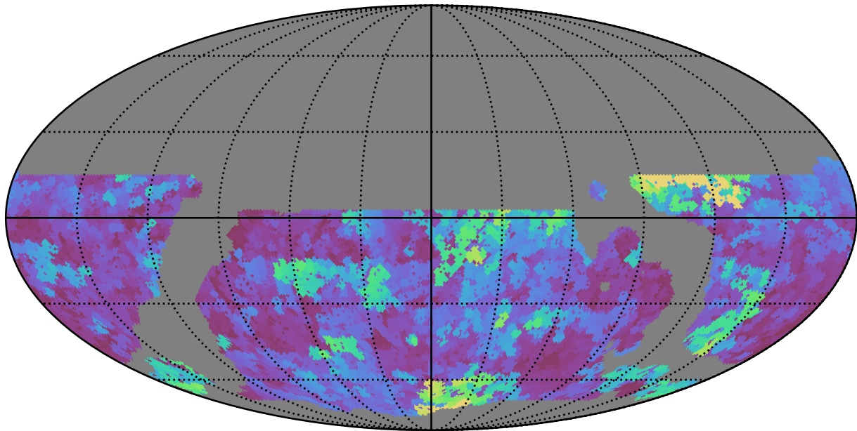
weather_cloudso20v3.4_10yrs WFD u band: Max seeingEff
