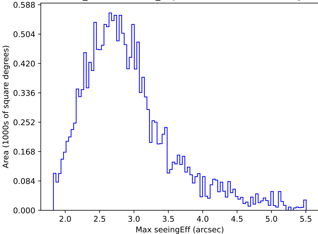
weather_cloudso20v3.4_10yrs WFD i band: Max seeingEff
