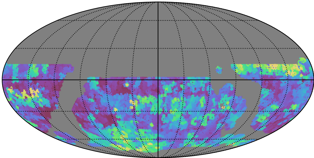
weather_cloudso20v3.4_10yrs WFD g band: Max seeingEff
