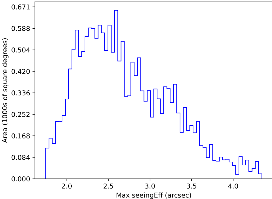
weather_cloudso20v3.4_10yrs WFD g band: Max seeingEff
