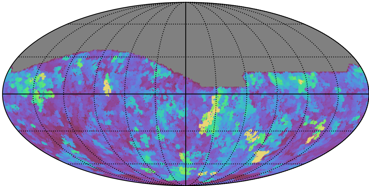
weather_cloudso20v3.4_10yrs All sky z band: Max seeingEff
