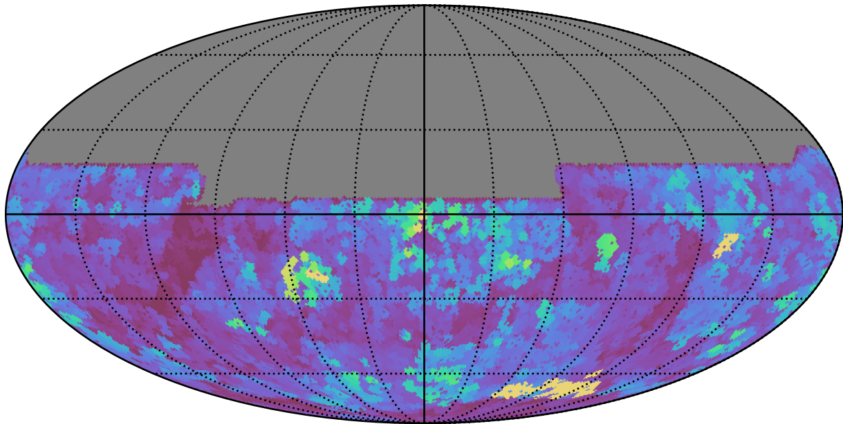
weather_cloudso20v3.4_10yrs All sky y band: Max seeingEff
