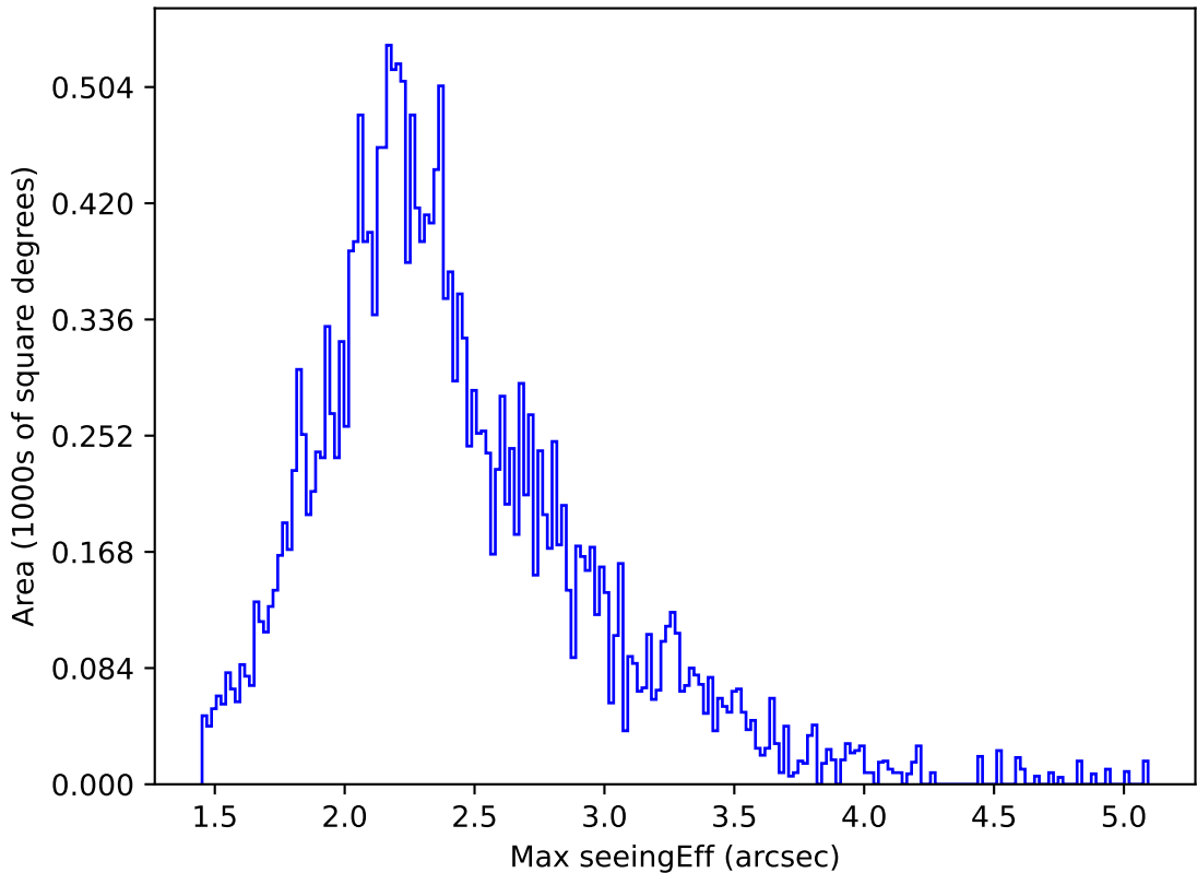
weather_cloudso20v3.4_10yrs All sky y band: Max seeingEff
