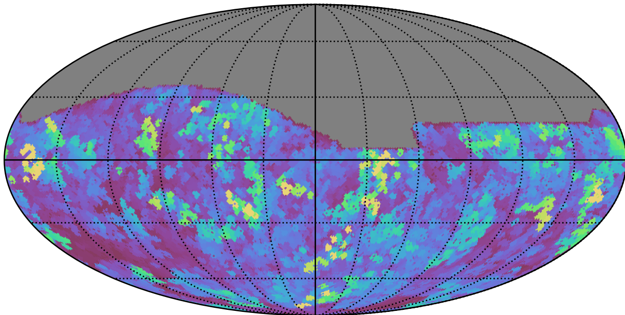
weather_cloudso20v3.4_10yrs All sky i band: Max seeingEff
