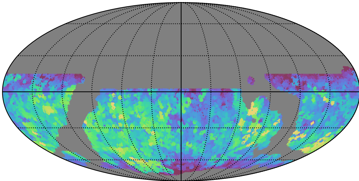
weather_cloudso20v3.4_10yrs WFD z band: Max saturation_mag
