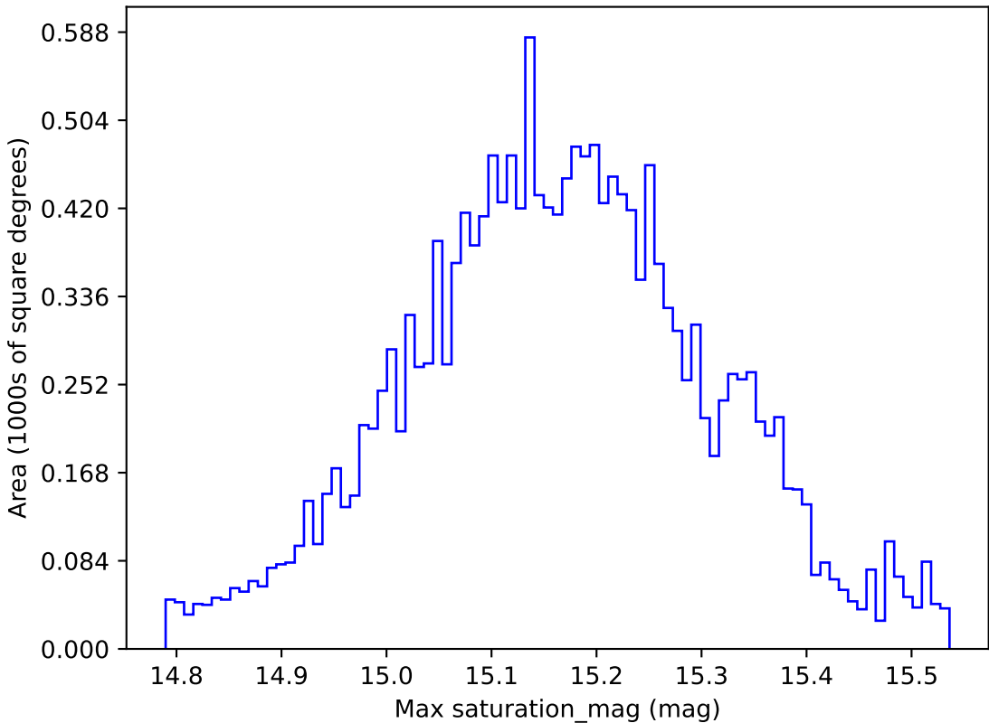
weather_cloudso20v3.4_10yrs WFD z band: Max saturation_mag
