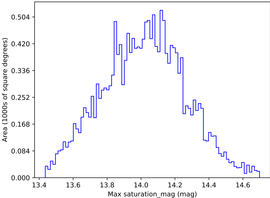
weather_cloudso20v3.4_10yrs WFD u band: Max saturation_mag
