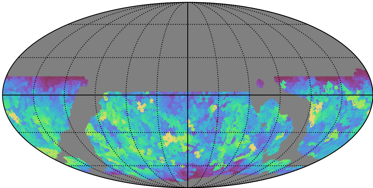
weather_cloudso20v3.4_10yrs WFD r band: Max saturation_mag
