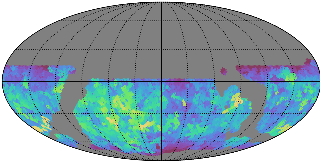
weather_cloudso20v3.4_10yrs WFD i band: Max saturation_mag
