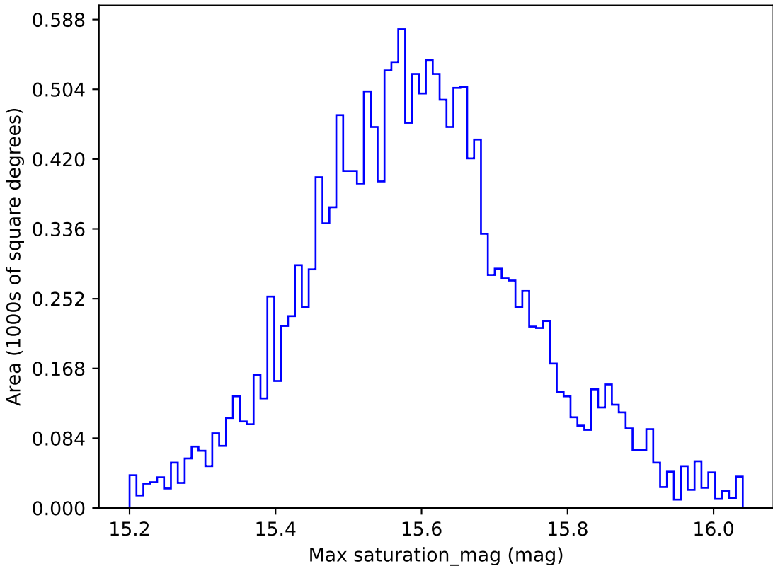
weather_cloudso20v3.4_10yrs WFD i band: Max saturation_mag
