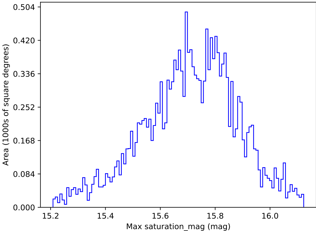
weather_cloudso20v3.4_10yrs WFD g band: Max saturation_mag
