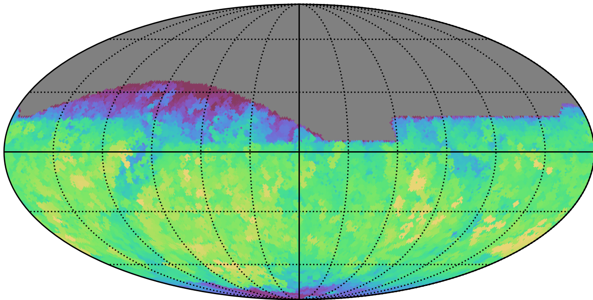
weather_cloudso20v3.4_10yrs All sky z band: Max saturation_mag
