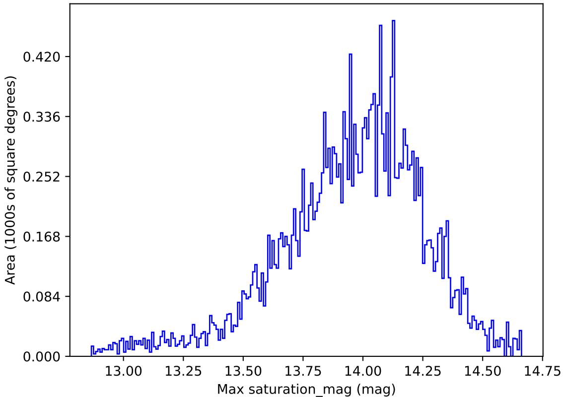
weather_cloudso20v3.4_10yrs All sky u band: Max saturation_mag
