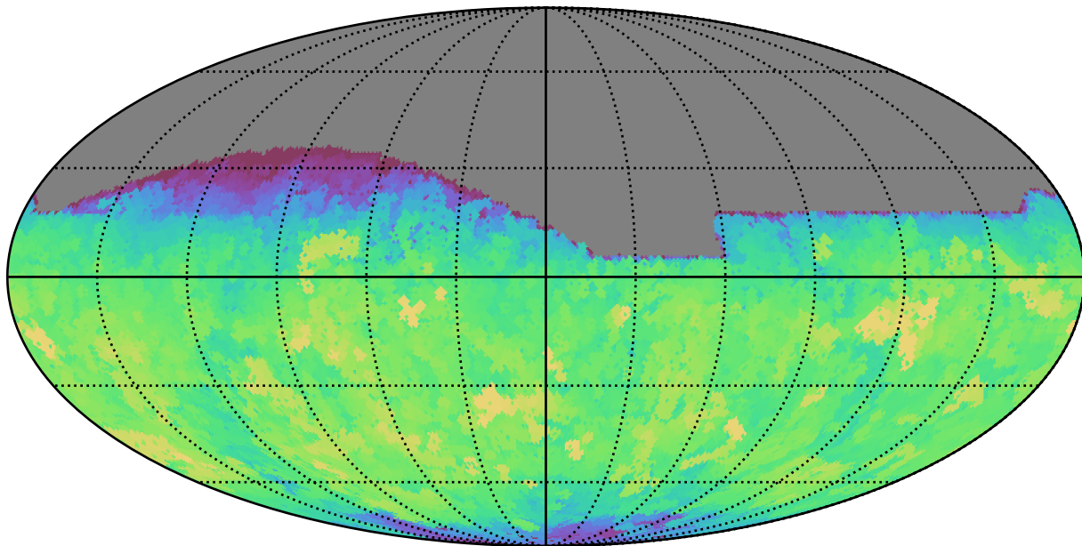
weather_cloudso20v3.4_10yrs All sky r band: Max saturation_mag
