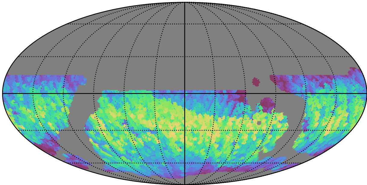
weather_cloudso20v3.4_10yrs WFD z band: Max normairmass
