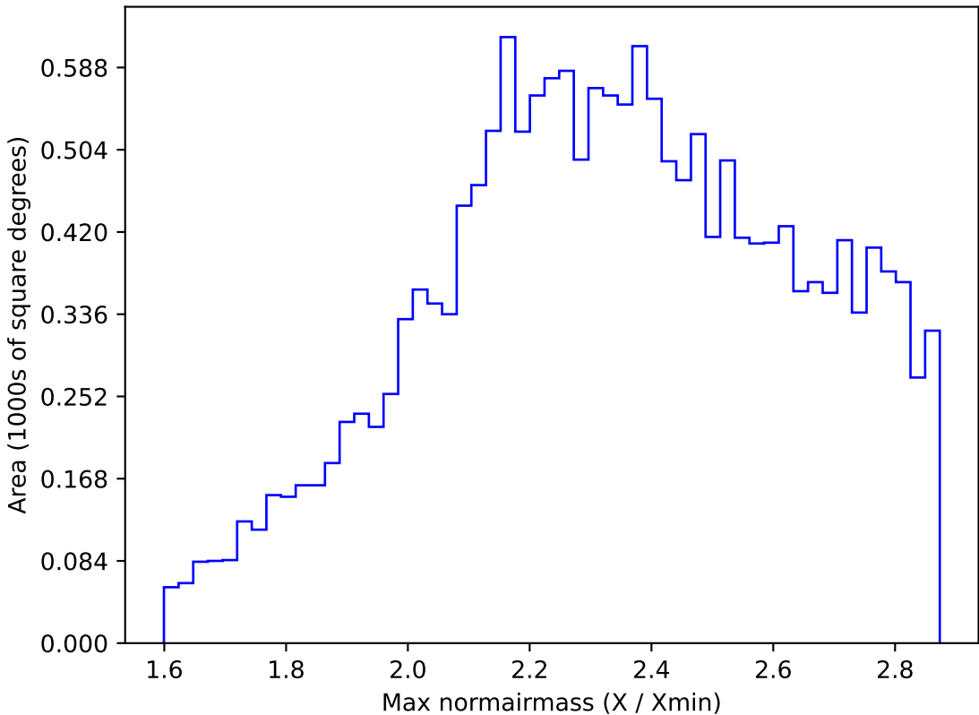
weather_cloudso20v3.4_10yrs WFD z band: Max normairmass
