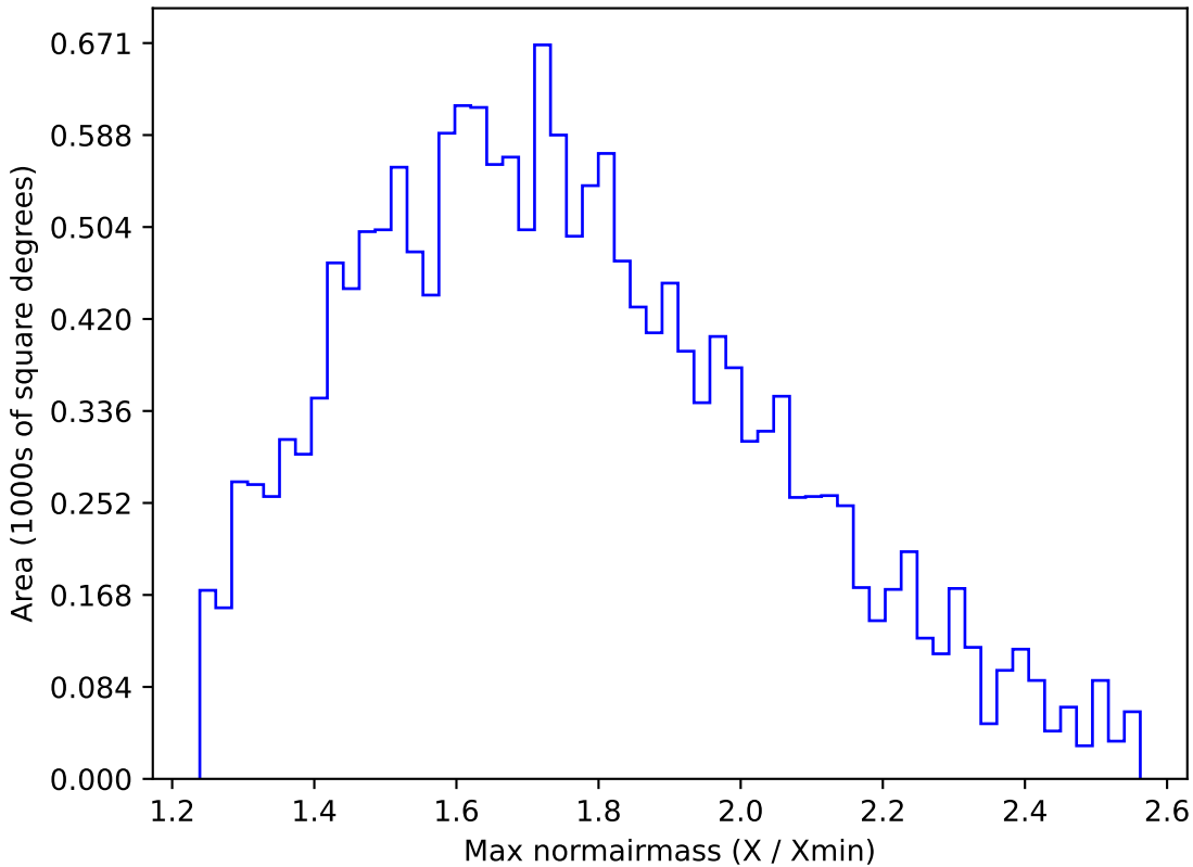
weather_cloudso20v3.4_10yrs WFD u band: Max normairmass
