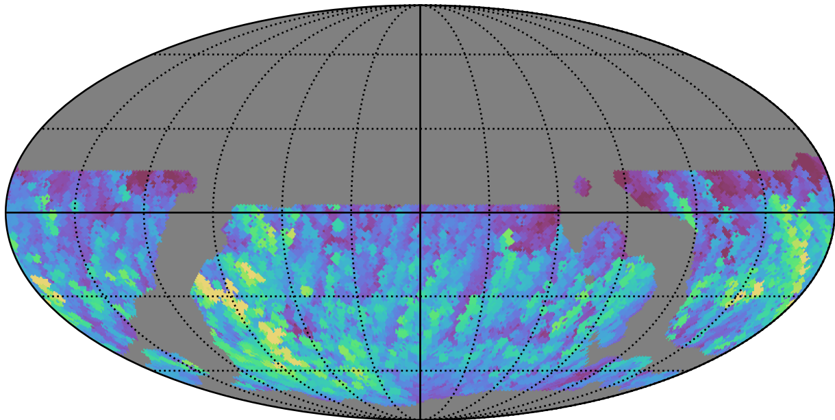
weather_cloudso20v3.4_10yrs WFD g band: Max normairmass
