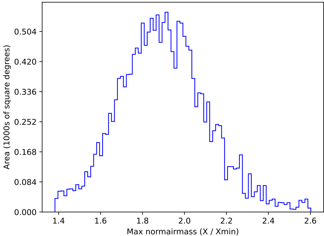
weather_cloudso20v3.4_10yrs WFD g band: Max normairmass
