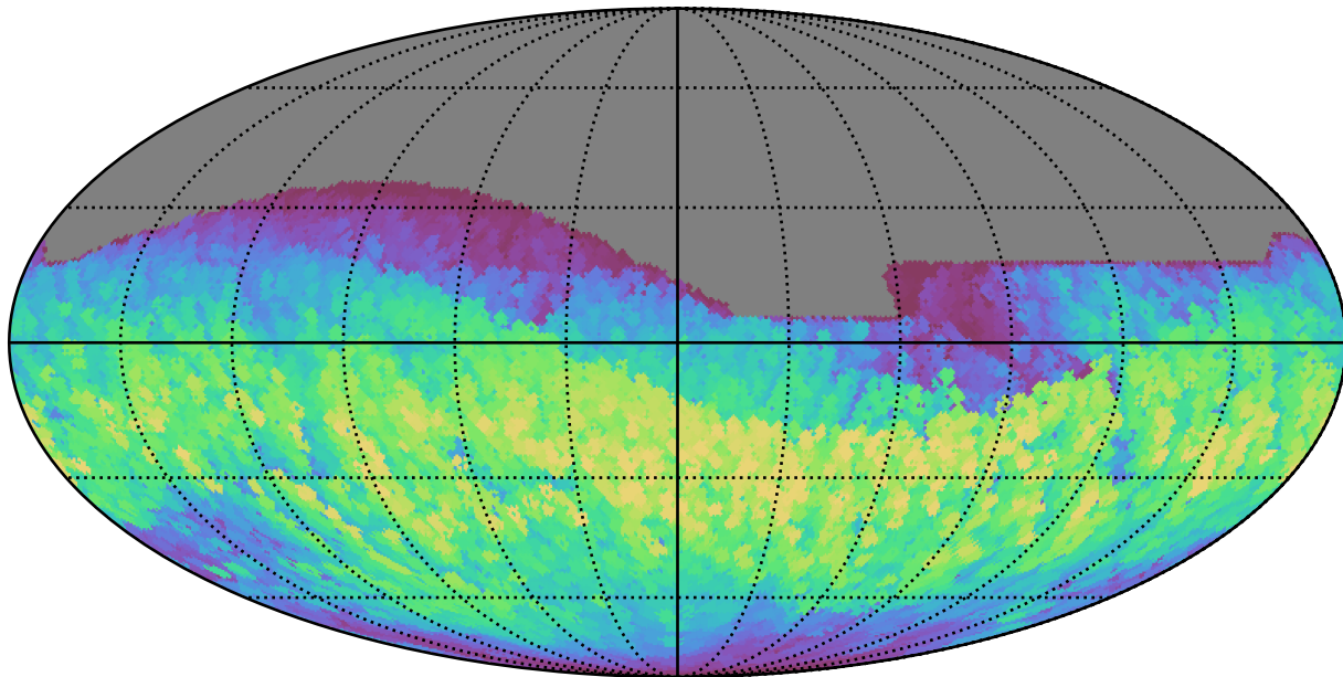
weather_cloudso20v3.4_10yrs All sky z band: Max normairmass
