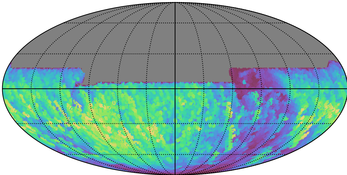
weather_cloudso20v3.4_10yrs All sky y band: Max normairmass
