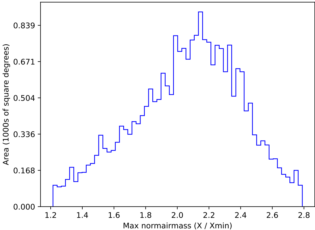
weather_cloudso20v3.4_10yrs All sky y band: Max normairmass
