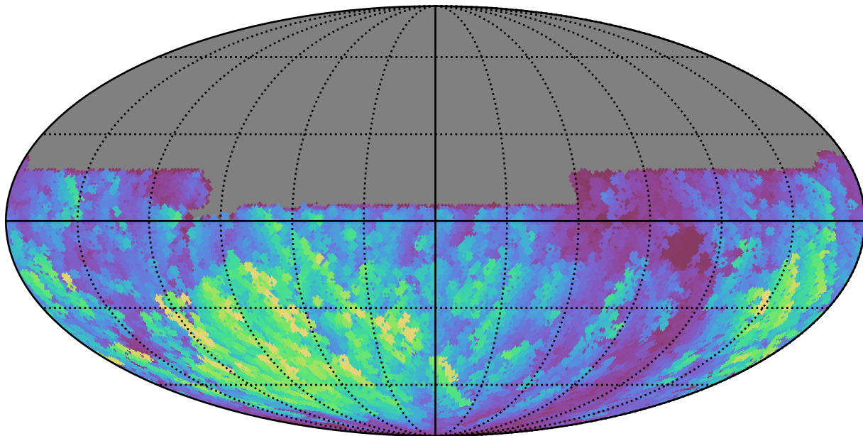
weather_cloudso20v3.4_10yrs All sky u band: Max normairmass
