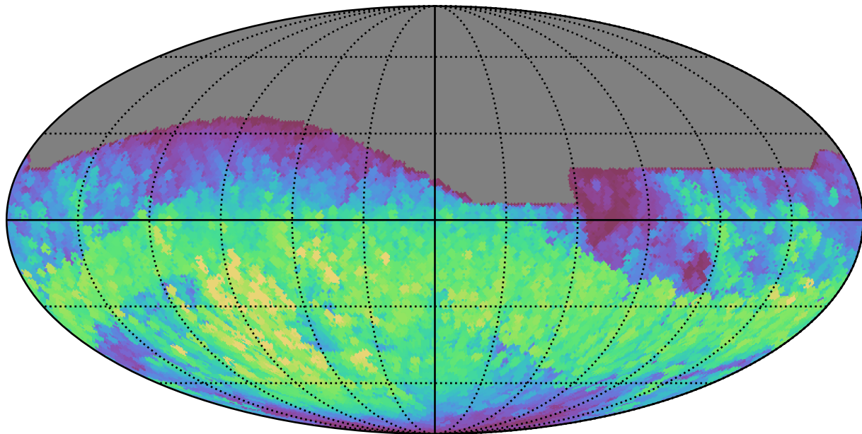
weather_cloudso20v3.4_10yrs All sky r band: Max normairmass
