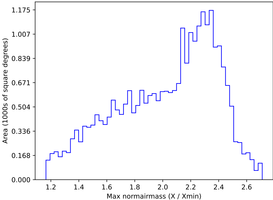
weather_cloudso20v3.4_10yrs All sky r band: Max normairmass
