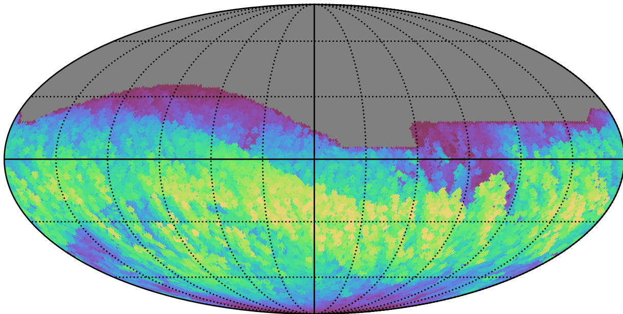
weather_cloudso20v3.4_10yrs All sky i band: Max normairmass
