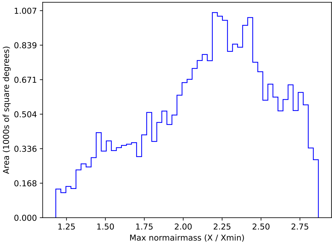
weather_cloudso20v3.4_10yrs All sky i band: Max normairmass
