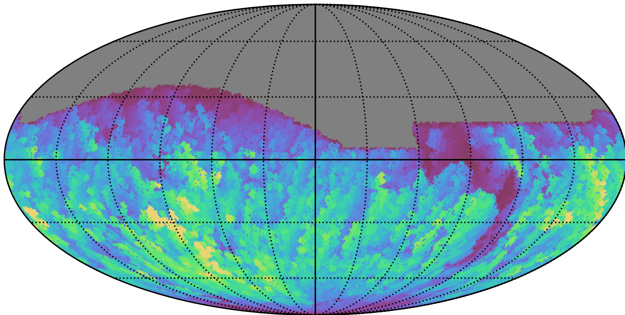
weather_cloudso20v3.4_10yrs All sky g band: Max normairmass
