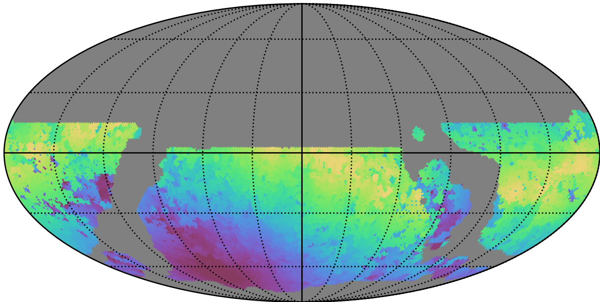
weather_cloudso20v3.4_10yrs WFD y band: Max moonDistance
