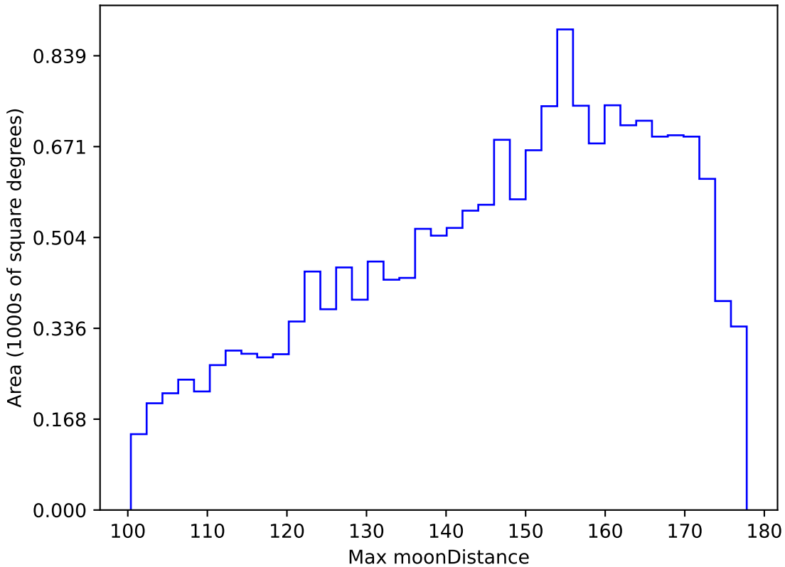
weather_cloudso20v3.4_10yrs WFD y band: Max moonDistance
