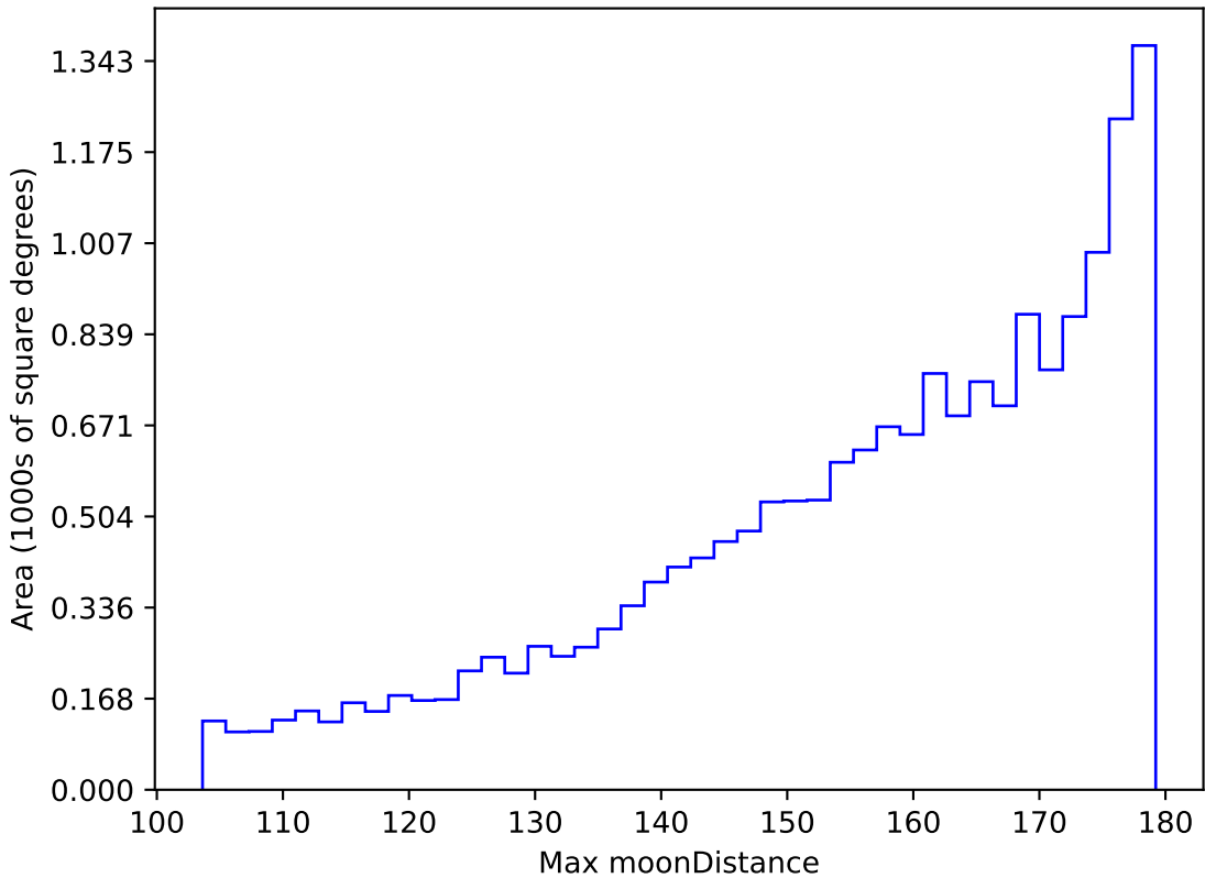
weather_cloudso20v3.4_10yrs WFD i band: Max moonDistance
