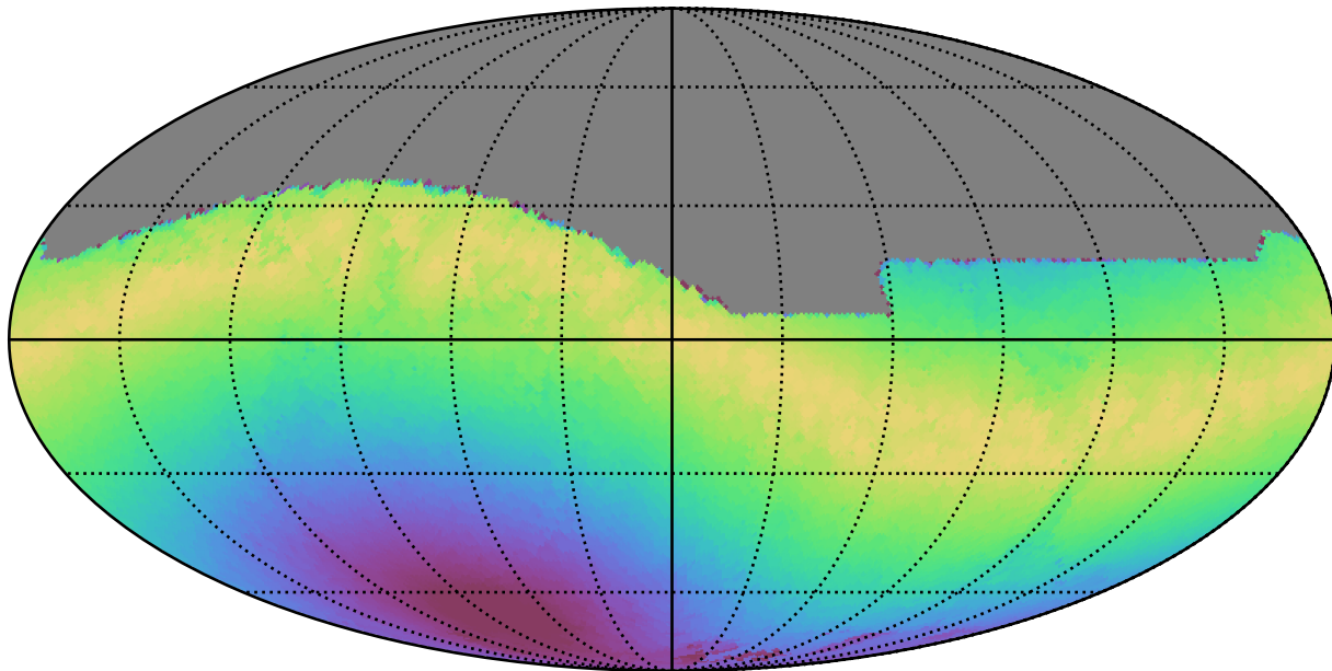
weather_cloudso20v3.4_10yrs All sky i band: Max moonDistance
