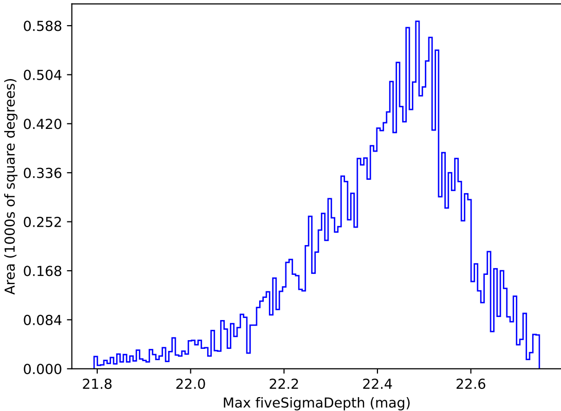
weather_cloudso20v3.4_10yrs Yr 1 y band: Max fiveSigmaDepth
