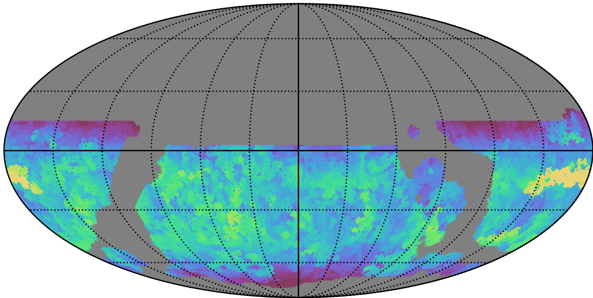
weather_cloudso20v3.4_10yrs WFD y band: Max fiveSigmaDepth
